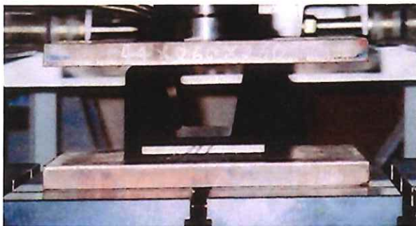
【圧縮テスト】 コメント：室温25℃
